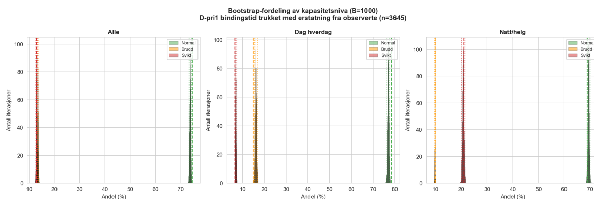
Figur 8.4: Bootstrap-fordeling av kapasitetsnivå ( B = 1\,000 ). Stiplet linje: punktestimat (median-imputert). Punkttert linje: 95 % CI-grenser.
